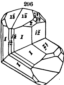
Manganite.
